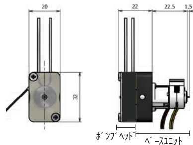
外観図
